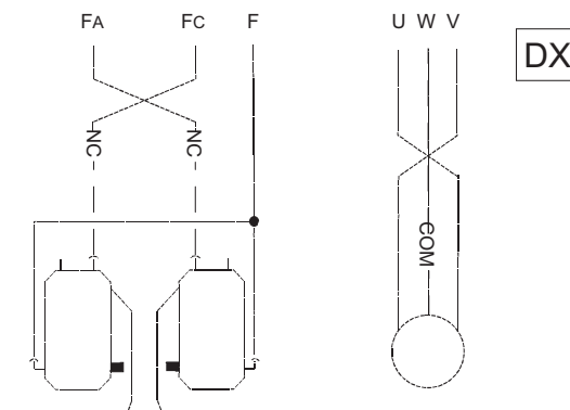
Блок микровыключателей
