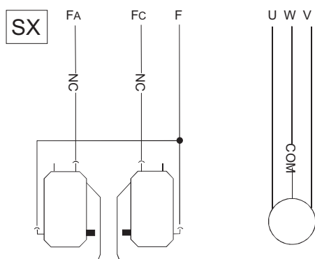
Блок микровыключателей
